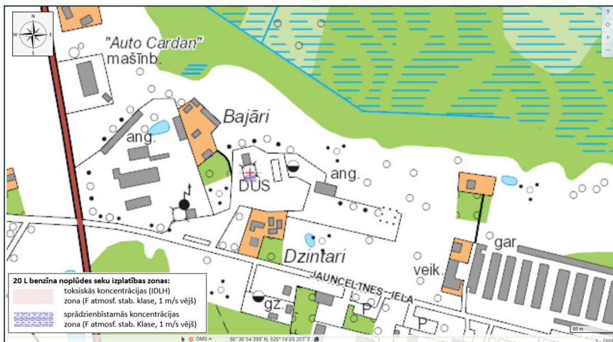
4.1. att. Toksiskās un sprādzienbīstamās koncentrācijas izplatības zonas 20 L noplūduša benzīna gadījumā (bez degšanas)
