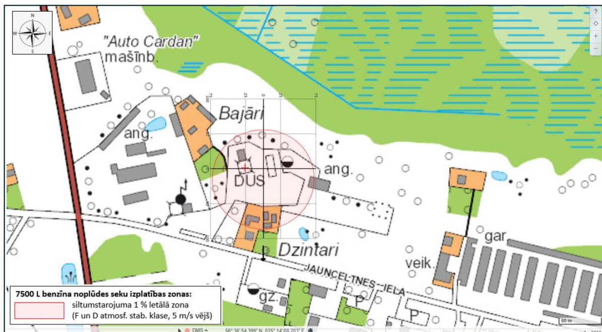
4.5. att. Siltumstarojuma izplatības zona 7500 L noplūduša benzīna gadījumā (ar degšanu)
