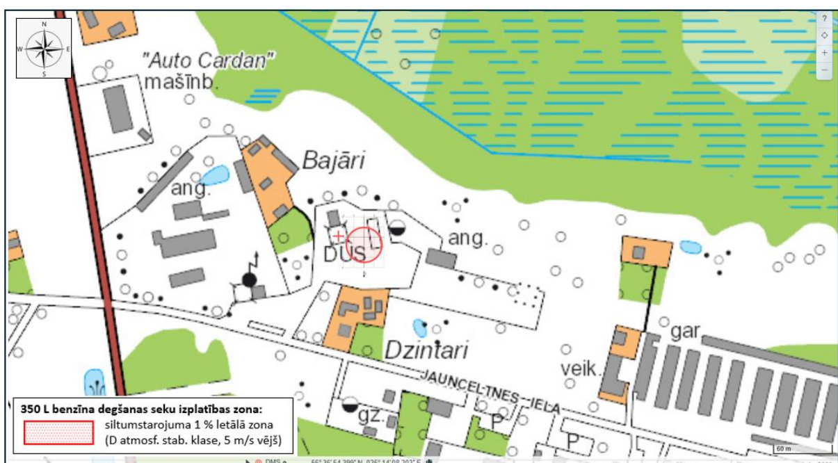
4.3. att. Siltumstarojuma izplatības zona 350 L noplūduša benzīna gadījumā (ar degšanu)
