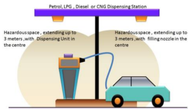
3.2. att. Sprādzienbīstamais zonējums automašīnas uzpildes laikā
