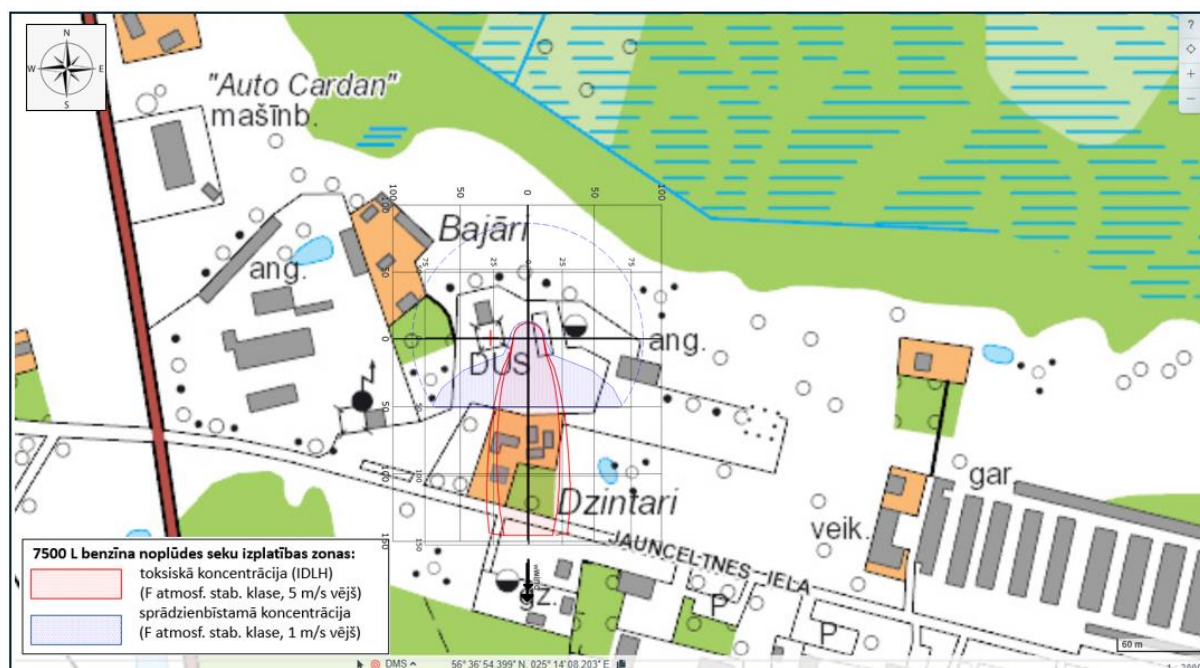
4.4. att. Toksiskās un sprādzienbīstamās koncentrācijas izplatības zonas 7500 L noplūduša benzīna gadījumā (bez degšanas)
