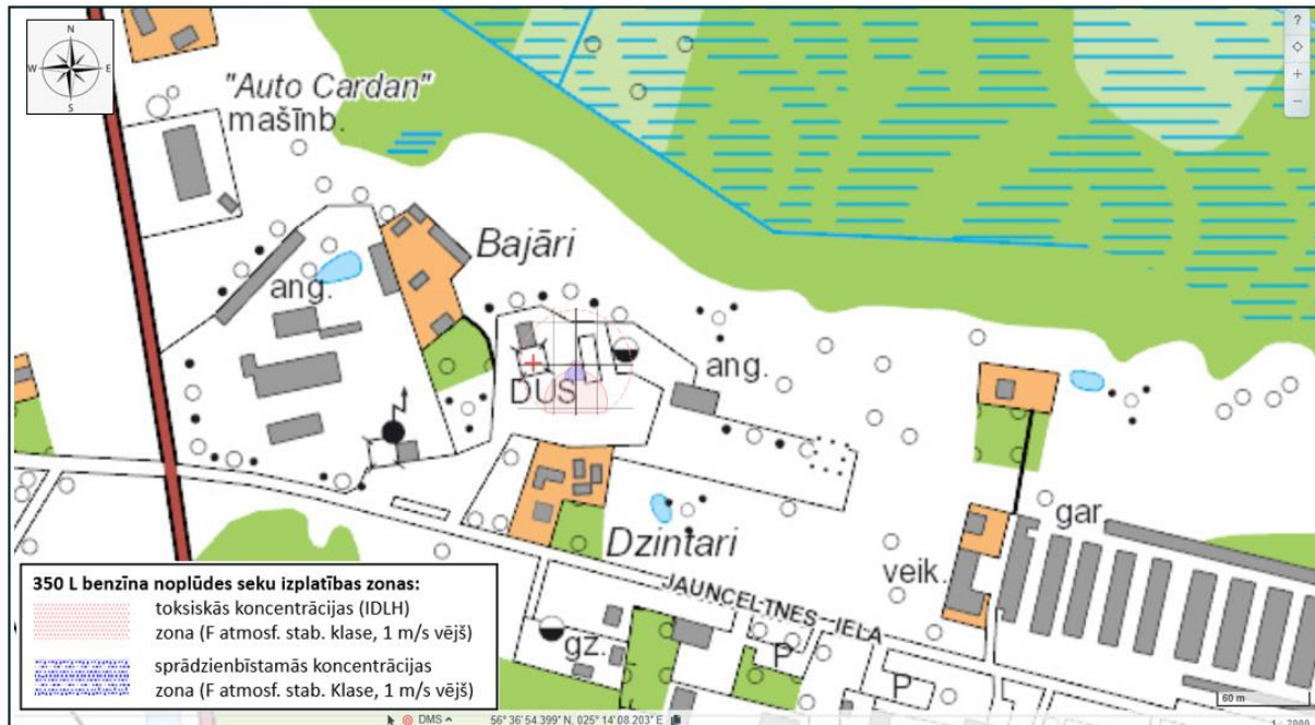
4.2. att. Toksiskās un sprādzienbīstamās koncentrācijas izplatības zonas 350 L noplūduša benzīna gadījumā (bez degšanas)
