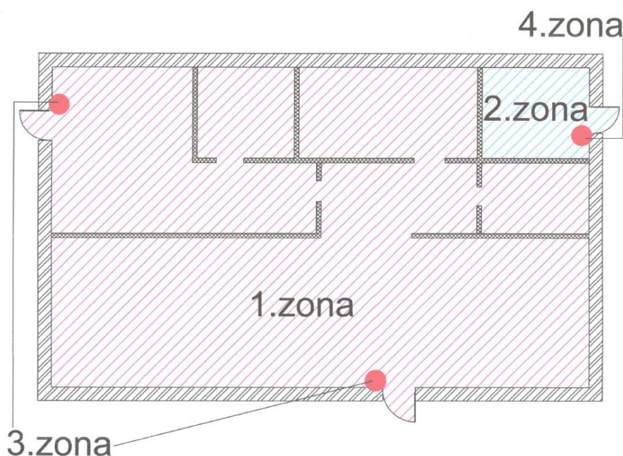
13.1. att. Uguns aizsargāto zonu sadalījums DUS "Skrīveri" ēkā
