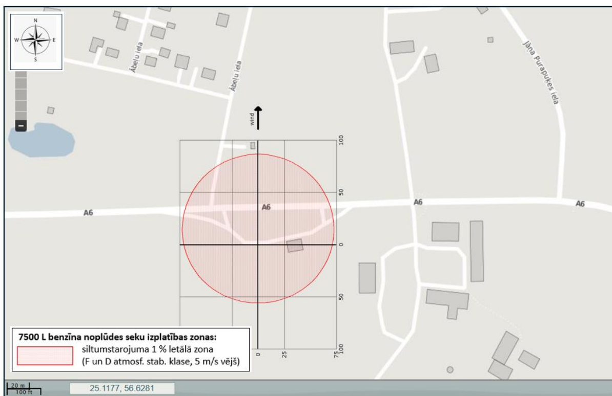
4.5. att. Siltumstarojuma izplatības zona 7500 L noplūduša benzīna gadījumā (ar degšanu)
