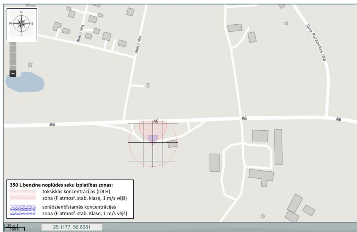
4.2. att. Toksiskās un sprādzienbīstamās koncentrācijas izplatības zonas 350 L noplūduša benzīna gadījumā (bez degšanas)
