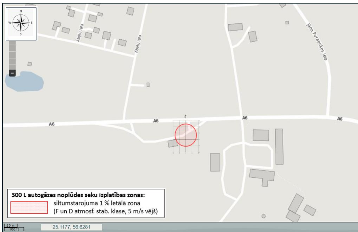
4.7. att. Siltumstarojuma izplatības zona 300 L noplūdušas autogāzes gadījumā (ar degšanu)
