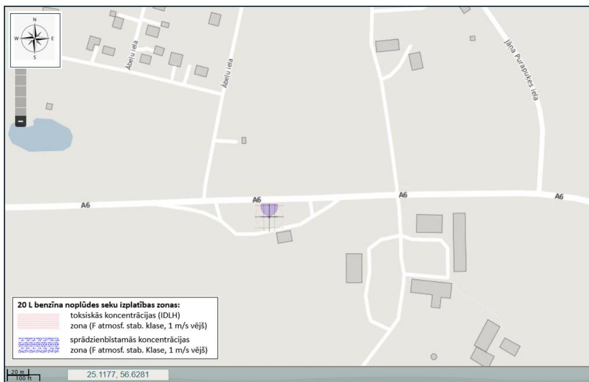
4.1. att. Toksiskās un sprādzienbīstamās koncentrācijas izplatības zonas 20 L noplūduša benzīna gadījumā (bez degšanas)
