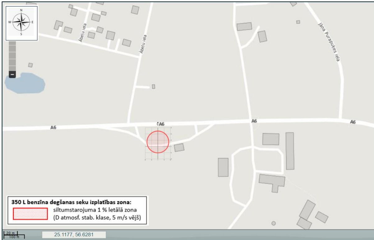
4.3. att. Siltumstarojuma izplatības zona 350 L noplūduša benzīna gadījumā (ar degšanu)
