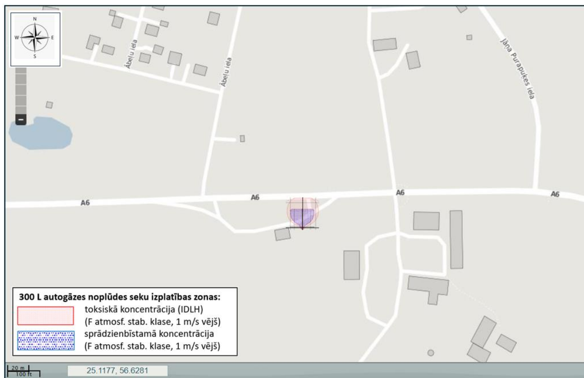
4.6. att. Toksiskās un sprādzienbīstamās koncentrācijas izplatības zonas 300 L noplūdušas autogāzes gadījumā (bez degšanas)
