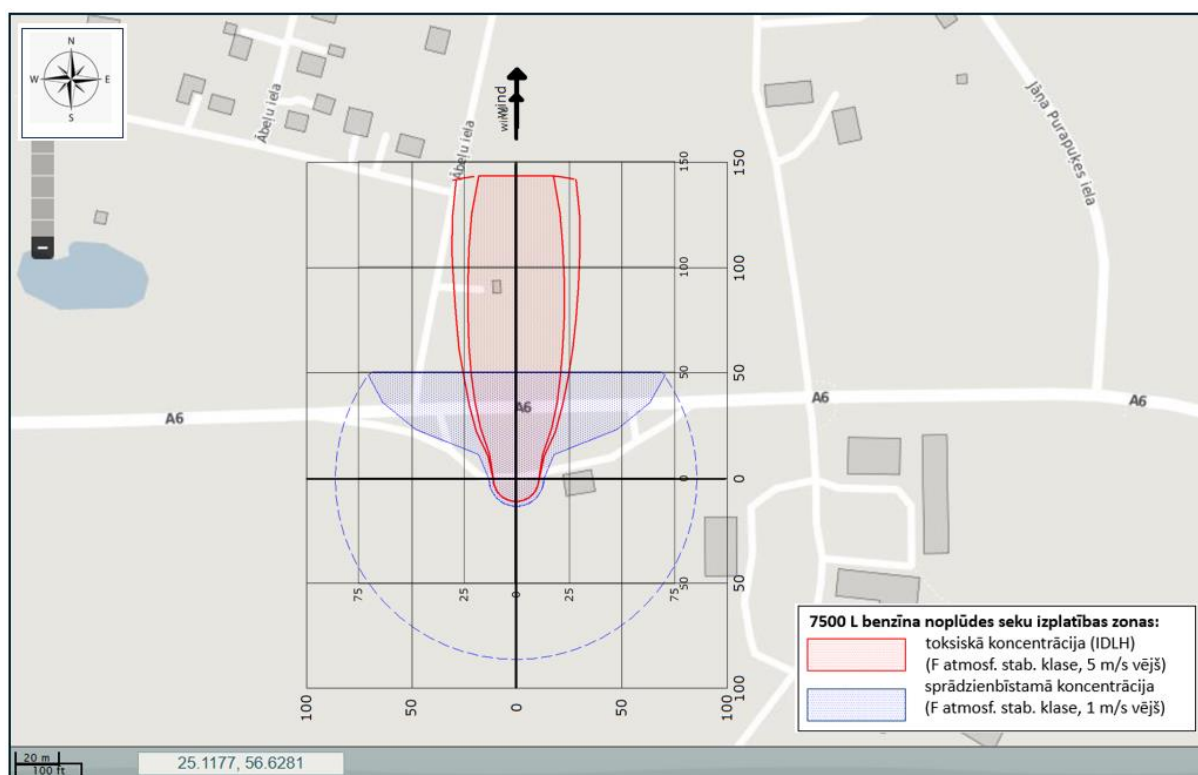
4.4. att. Toksiskās un sprādzienbīstamās koncentrācijas izplatības zonas 7500 L noplūduša benzīna gadījumā (bez degšanas)
